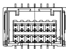
12-18極 12-18 CKT
