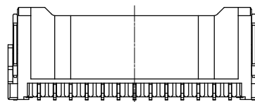
20-28極 20-28 CKT
