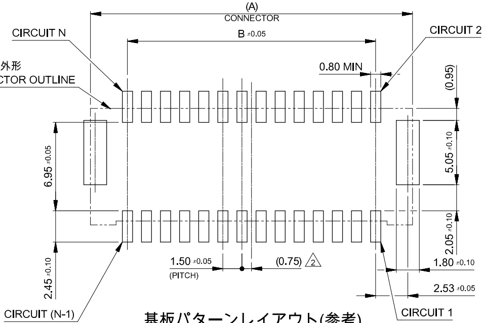
基板パターンレイアウト(参考) RECOMMENDED PCB PATTERN LAYOUT (REF.) (参考: メタルマスク厚さ 0.10mm, マスク開口率100%) (REFERENCE: METAL MASK THICKNESS 0.10MM, APERTURE RATIO 100%)
